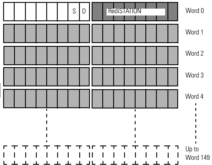
1747-SDN Module M1 File Data Table
